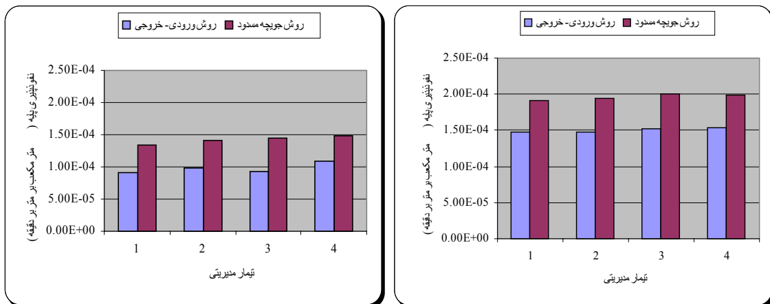
شکل ۱- مقادیر سرعت نفوذ پایه خاک در مدیریت‌های مختلف زراعی با دو روش اندازه‌گیری در ابتدای فصل رشد (راست) و اواسط فصل رشد (چپ)
